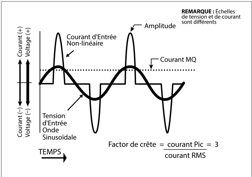
Fig. 4.2: Facteur de Crête élevé du courrant pris par l'Alimentation à Découpage
