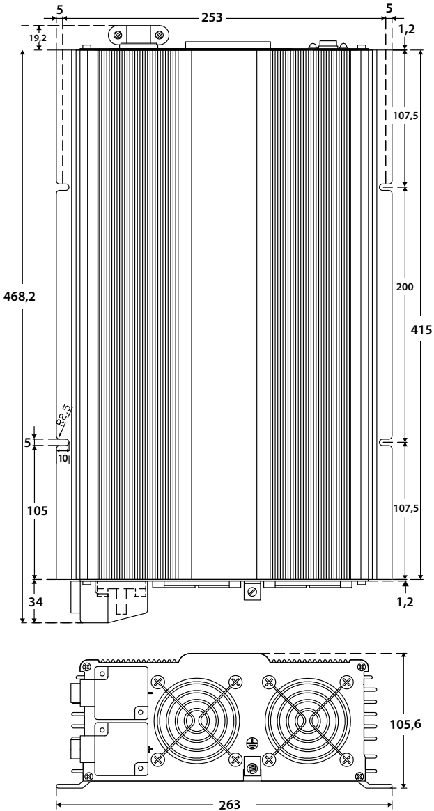
Fig. 8.1: Les Dimensions Générales et Rainures de Montages des PST-1500 et PST-2000 (NB: Dimensions en mm)
