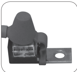
Fig. 3,11. CFBAR avec le fusible MRBF installé
