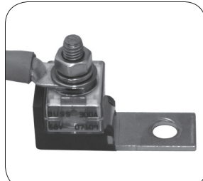
Fig 3,9. Fusible MRBF et câble positif fixé sur le CFBAR
